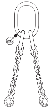
Kuva 14. Kettinkiraksi.
