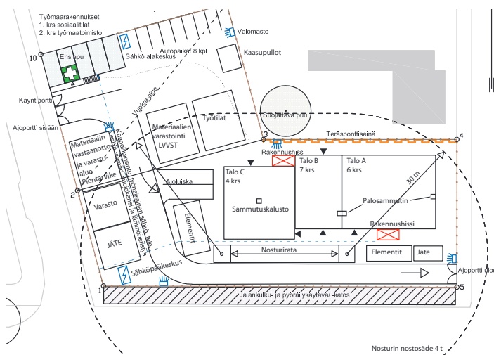
Kuva 5. Aluesuunnitelma.
