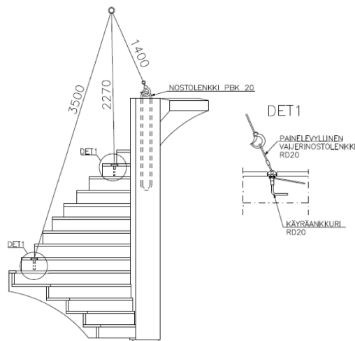
Kuva 33. Porrasvalmistajan ohje raksien pituudesta, nostokohdista ja nostolenkeistä. (Kuva: Lemminkäinen Betonituote Oy, asennusohje)
