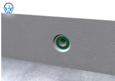
Kuva 13. Värikoodilla merkattu sisäkierrenostoankkuri. (Kuva: Peikko Finland Oy)
