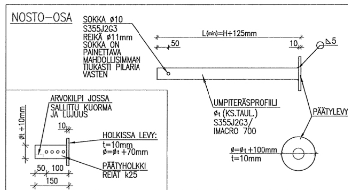
Kuva 26. Esimerkki pilarin nostoakselista.
