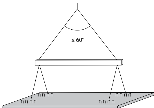
Kuva 31. Kuorilaatan nosto nostopalkkia käyttäen.
