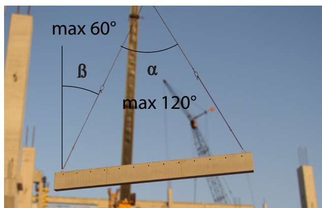
Kuva 16. Nostokulma beta ( \beta ) ei saa ylittää 60 astetta. Vastaavasti haarakulma alfa ( \alpha ) ei saa ylittää 120 astetta.
