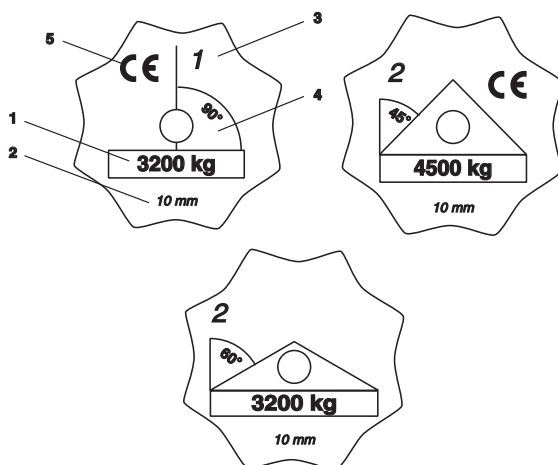
Kuva 15. Merkintälevyke.
