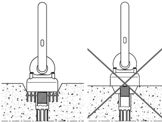
Kuva 22. Painelevyllisen nostolenkin asennus. (Kuvat: Peikko Finland Oy)
