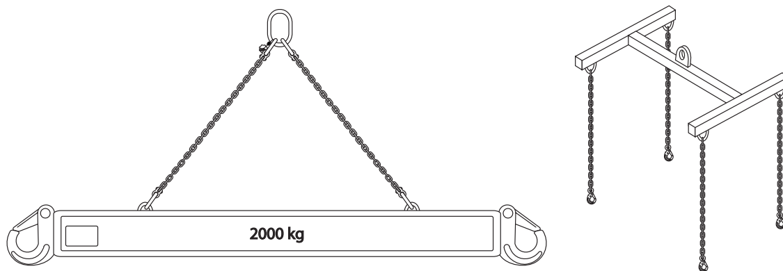
Kuva 19. Nostopalkkeja.
